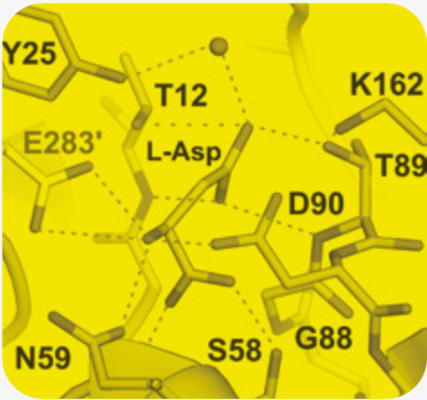
Struktura L-asparaginazy klasy pierwszej z wyodrębnionym miejscem aktywnym. Interakcje L-Asp w centrum katalitycznym L-asparaginazy klasy pierwszej.
