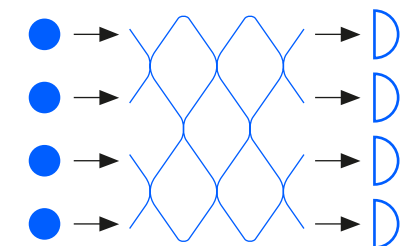
Obwód optyczny
